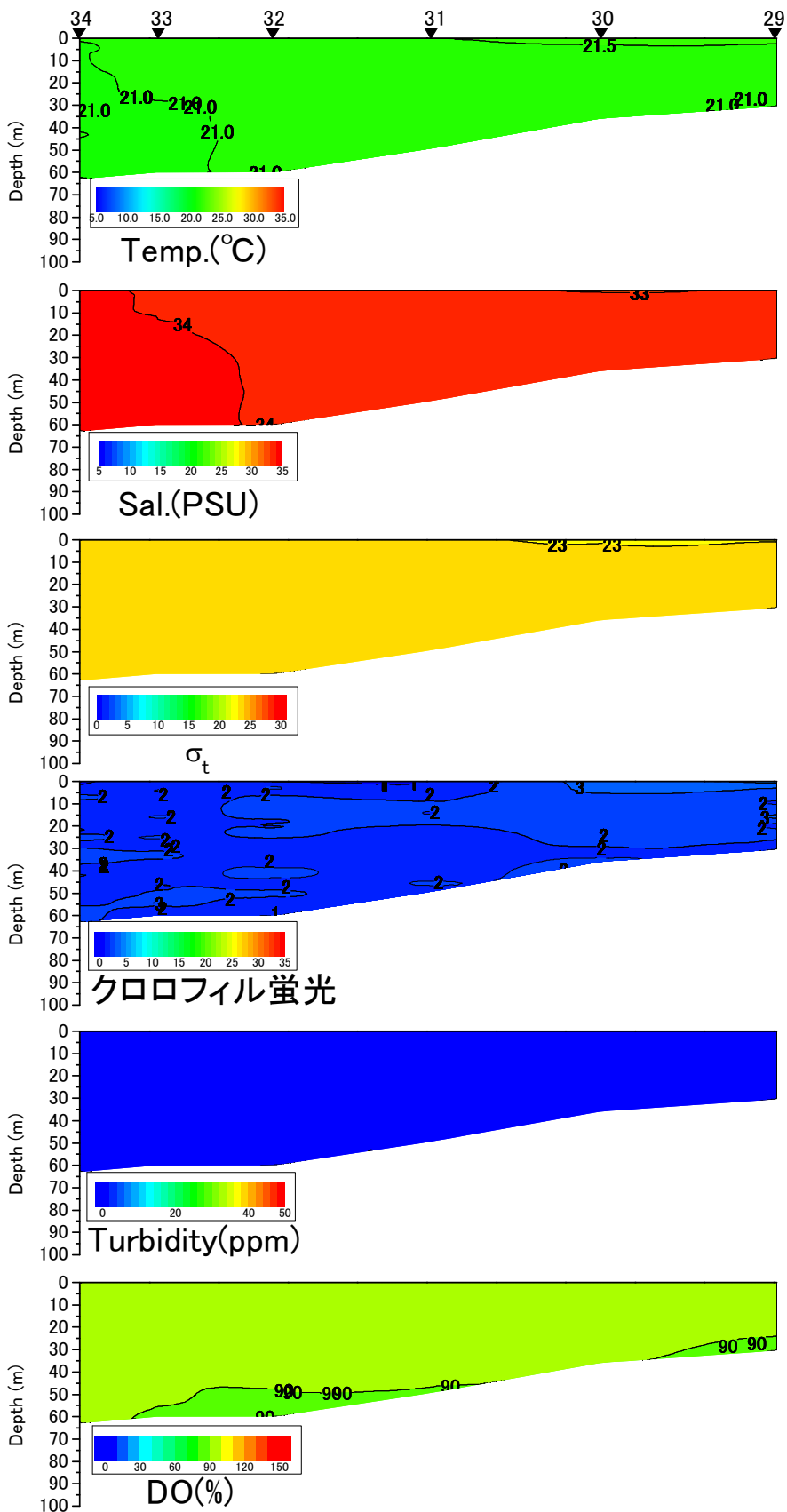
八代海西ラインの水温(°C)、塩分、密度( \sigma_t )、クロロフィル蛍光強度、濁度、溶存酸素飽和度(DO%)の鉛直面図(国土交通省の調査による) (2014年6月19日)
